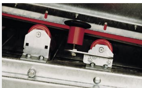
* Guide roller
